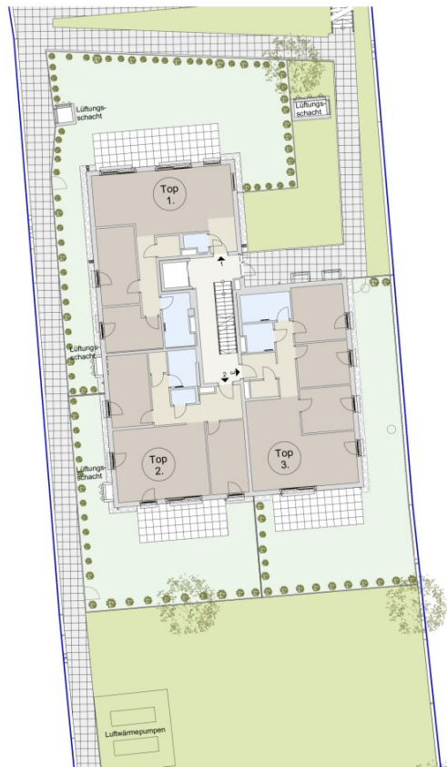
ERDGESCHOSS 1 : 200
