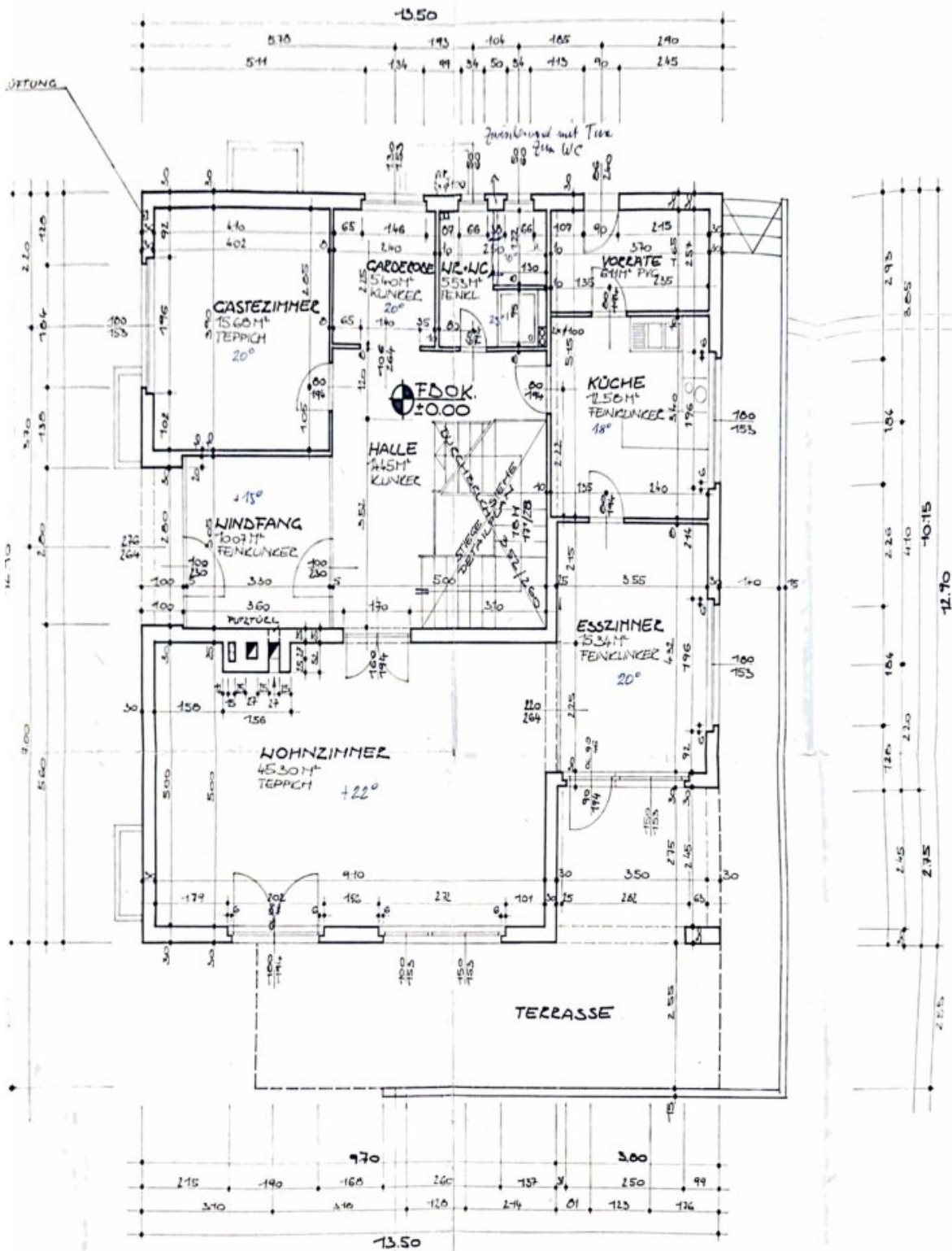
ERDGESCHOSS M 1:50
