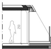
SCHNITT B
