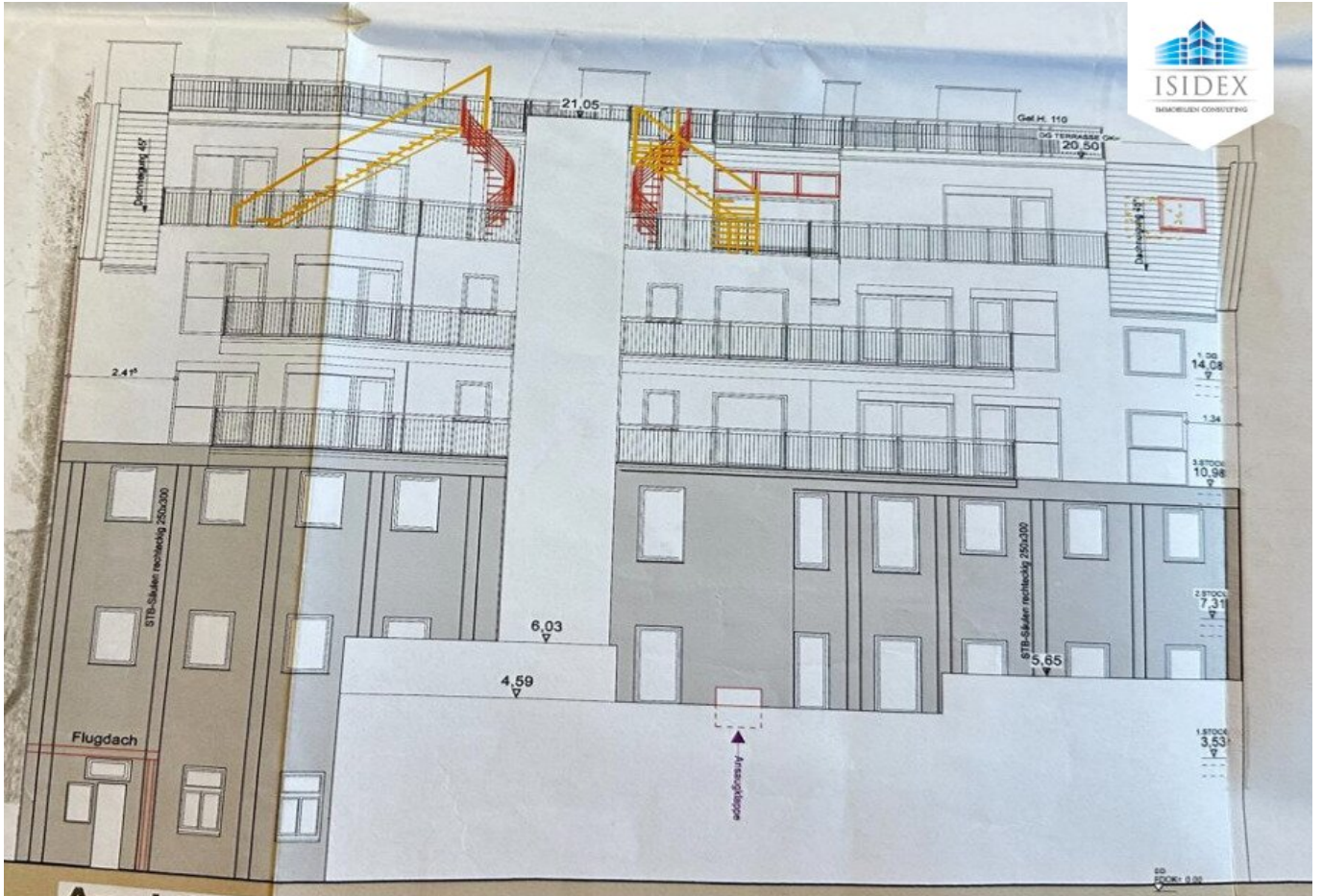
Ansicht Ost
