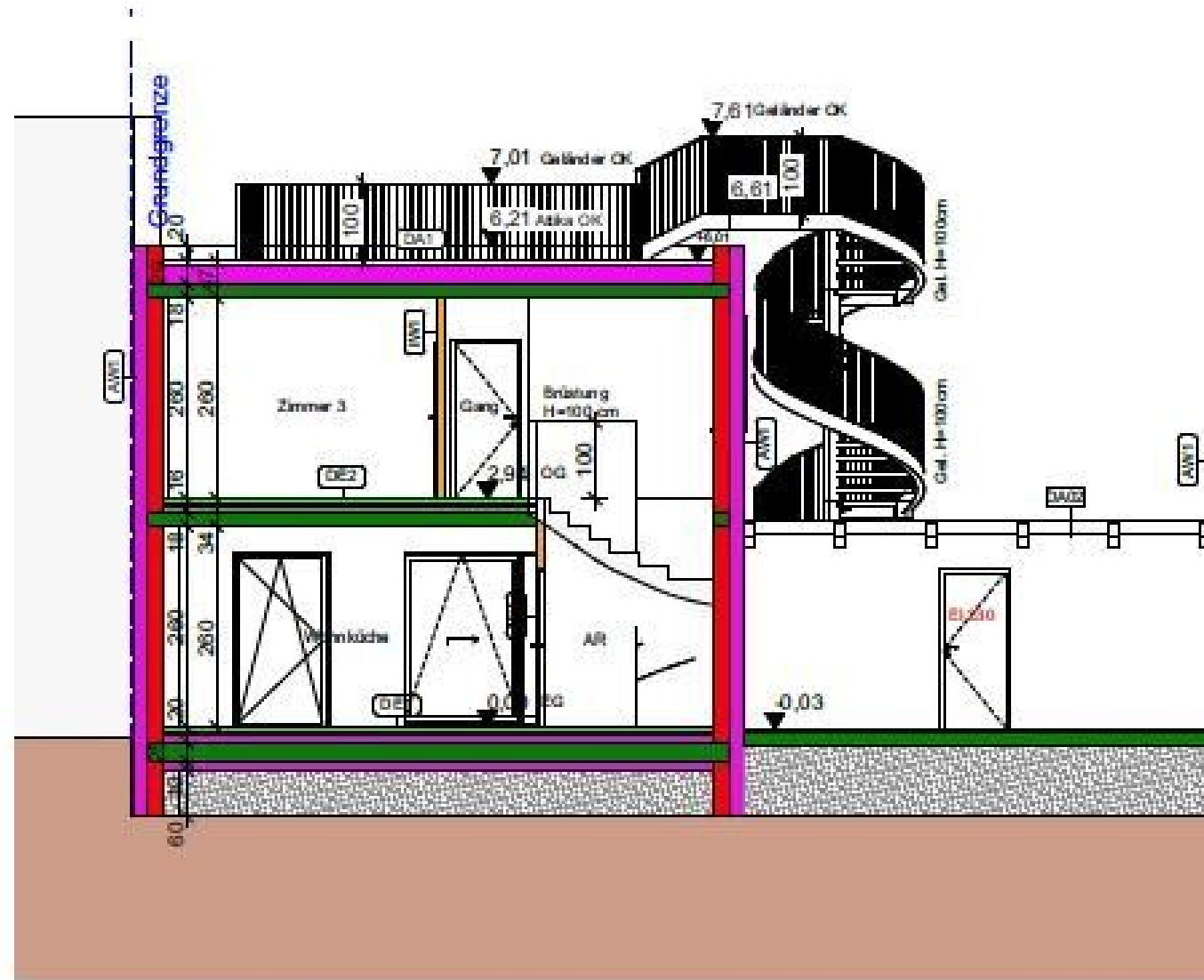
SCHNITT A-A M:100
