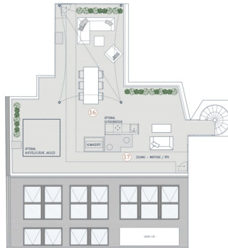
Dachterrasse
