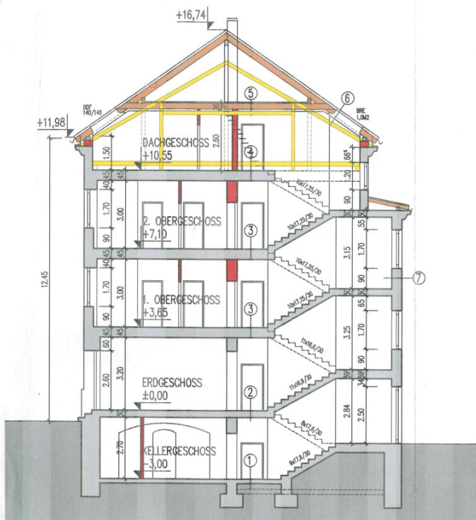
SCHNITT A-A
