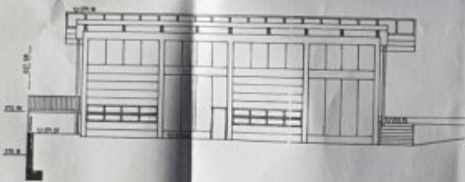
ANSICHT NW
