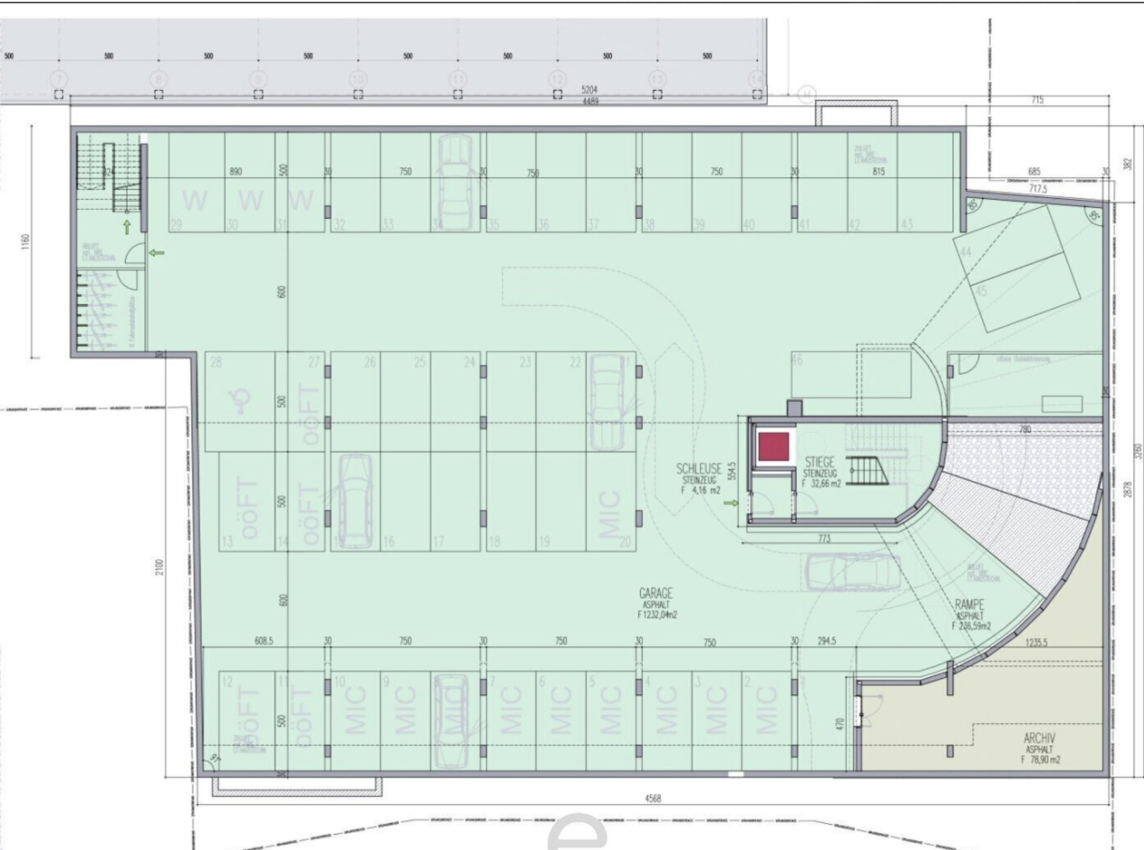
Am Winterhafen 4 - BT2 Neubau - 1.UIG - M 1:150
