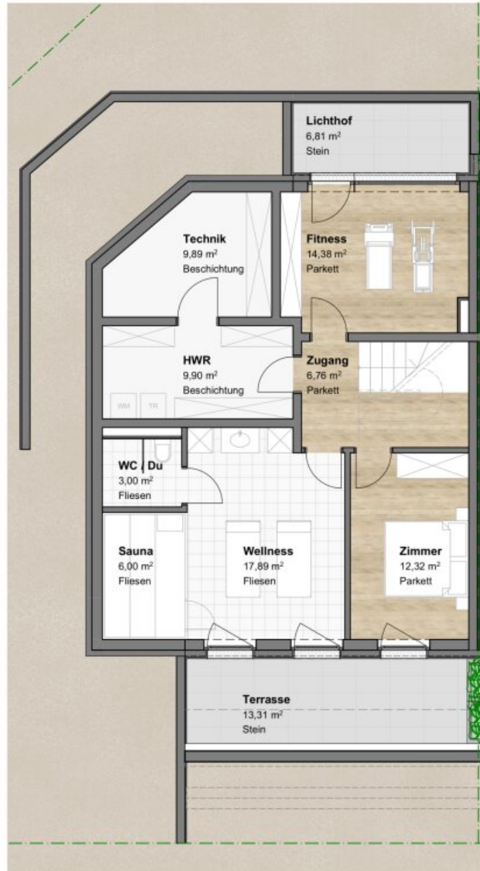
Grundriss Untergeschoß 1:100
