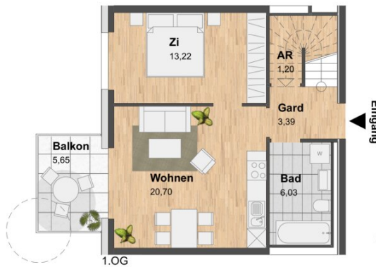
Grundriss 1:100
