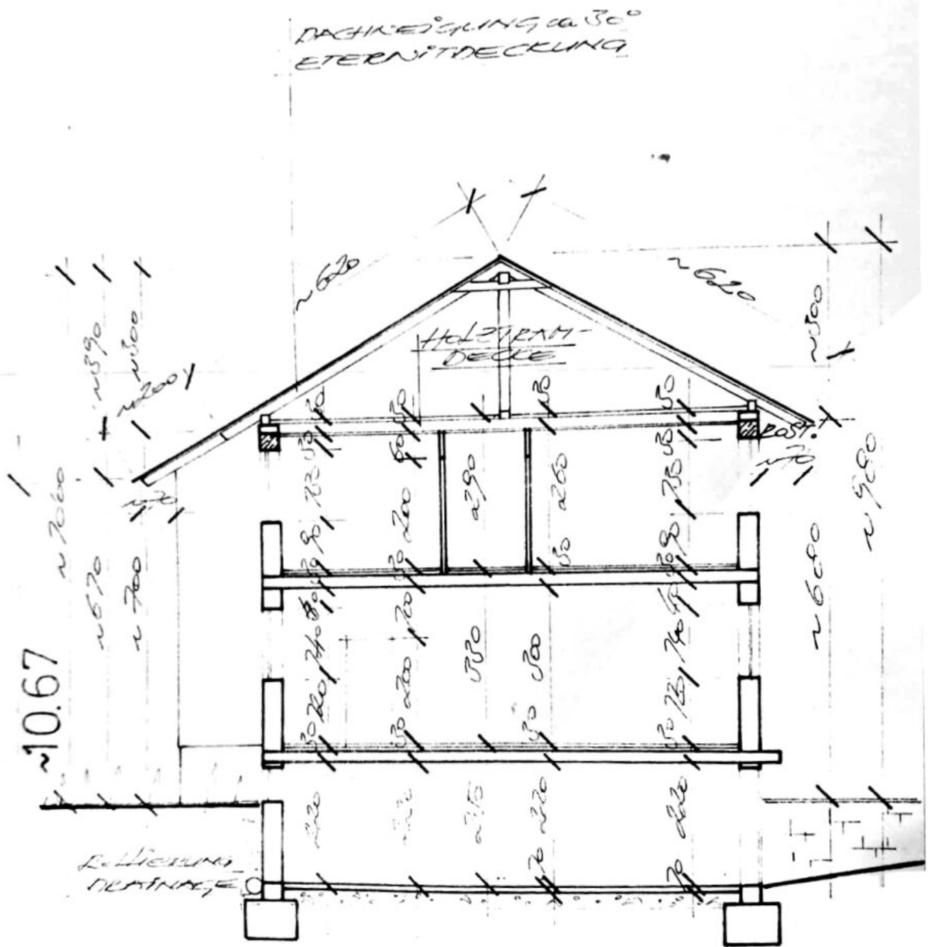
SCHNITT A-A
