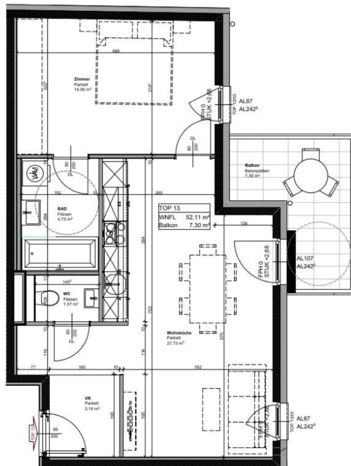
GRUNDRISS 1.OBERGESCHOSS
