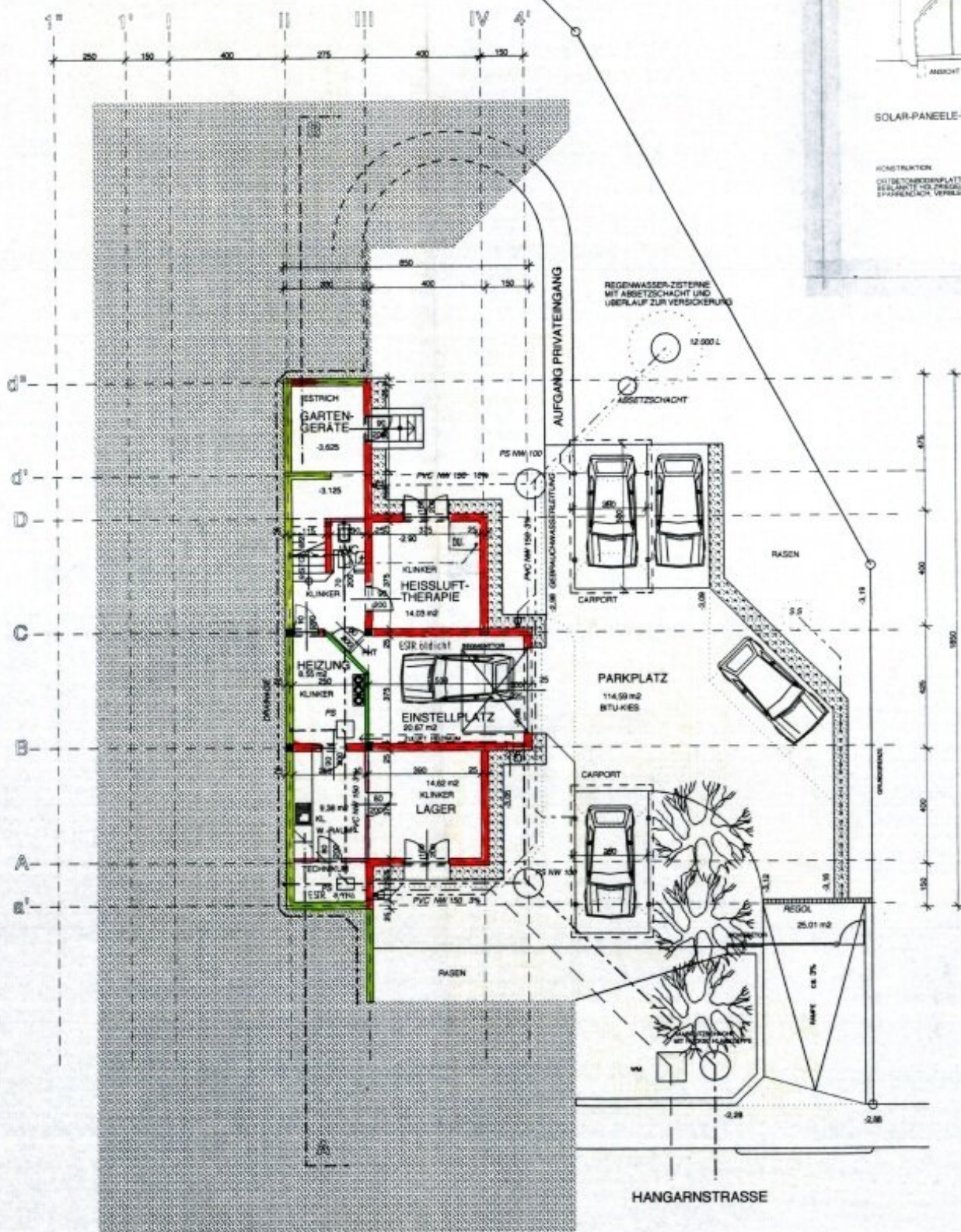
GRUNDRISS UNTERGESCHOSS
