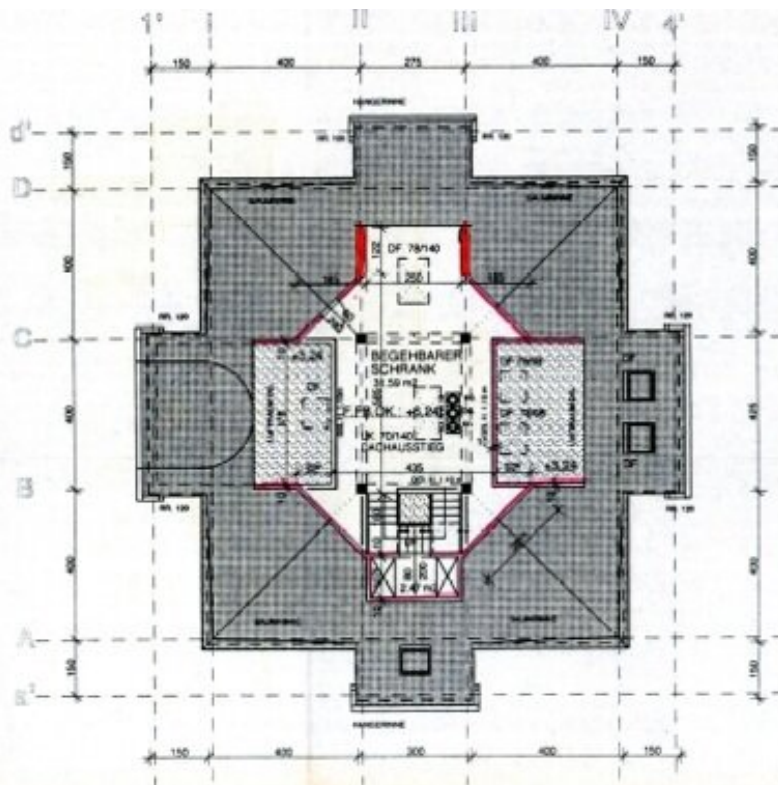
GRUNDRISS EMPORE (BEGEHBARER SCHRANK)
