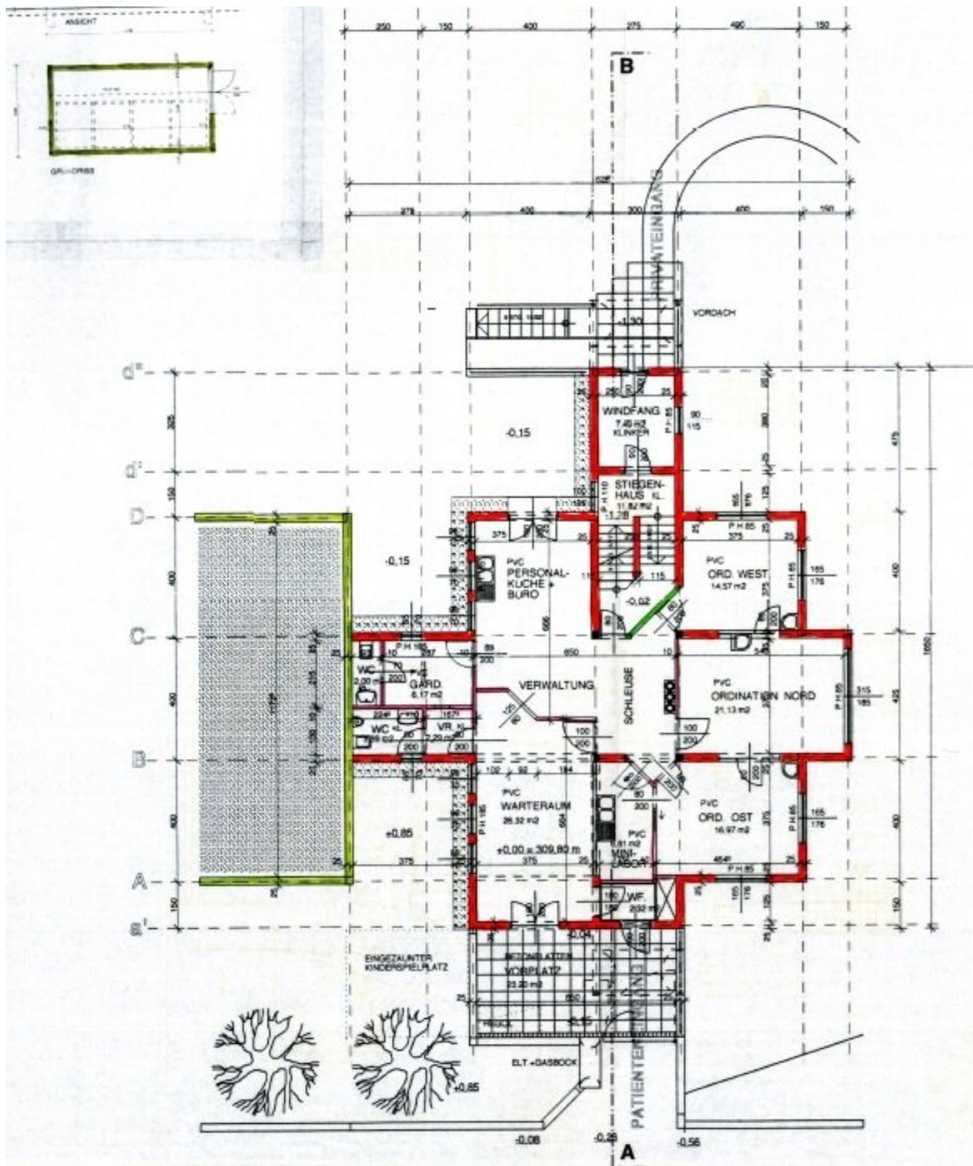
GRUNDRISS ERDGESCHOSS
