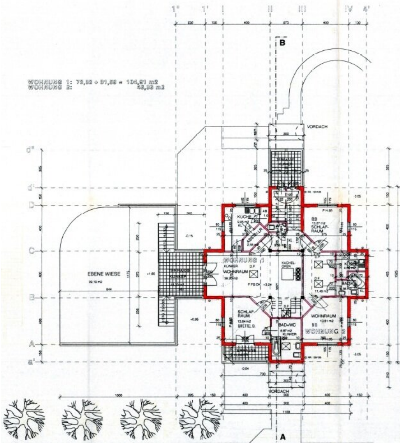
GRUNDRISS OBERGESCHOSS
