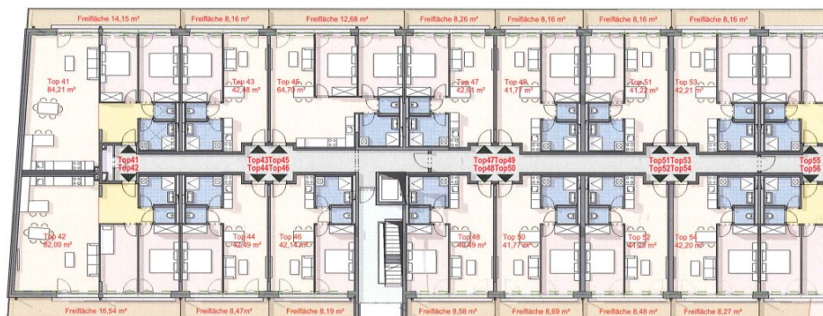
2.OBERGESCHOSS M 1:200
