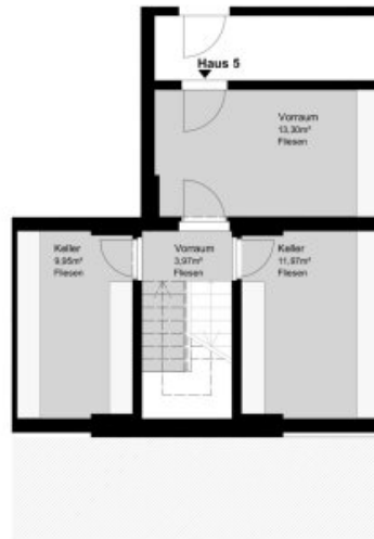
HAUS 5 - KELLERGEESCHOSS / TIEFGARAGE
