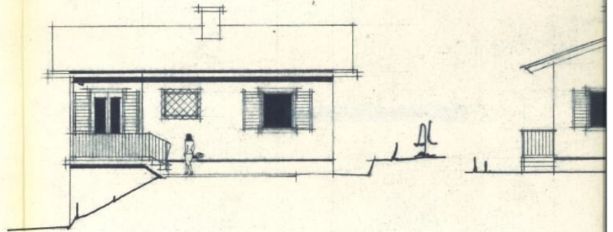
SÜD - OST - ANSICHT
