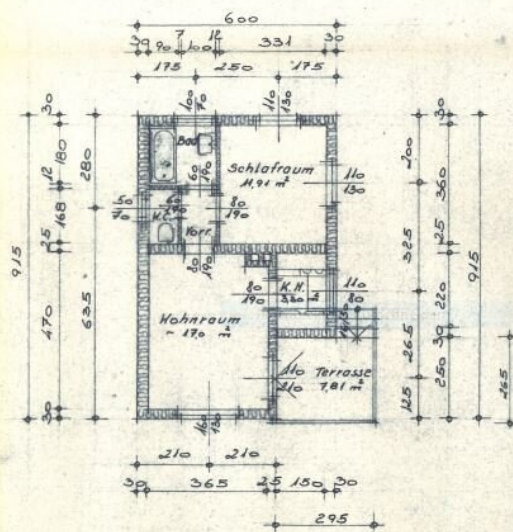
ERDGESCHOSS
