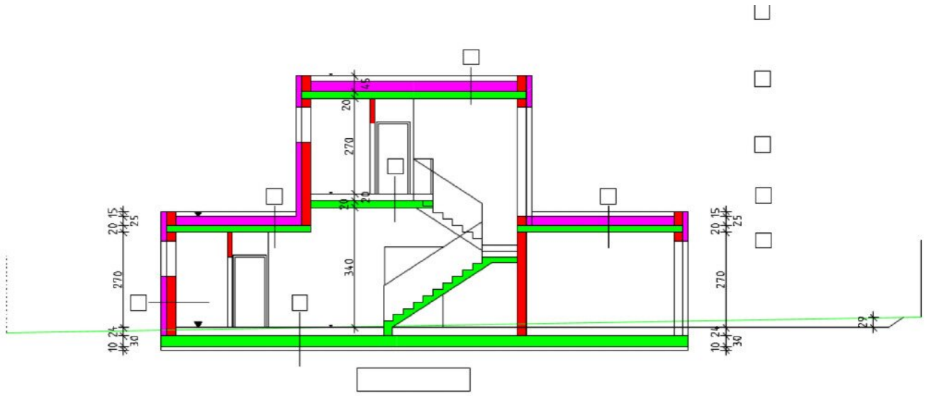
SCHNITT A-A
