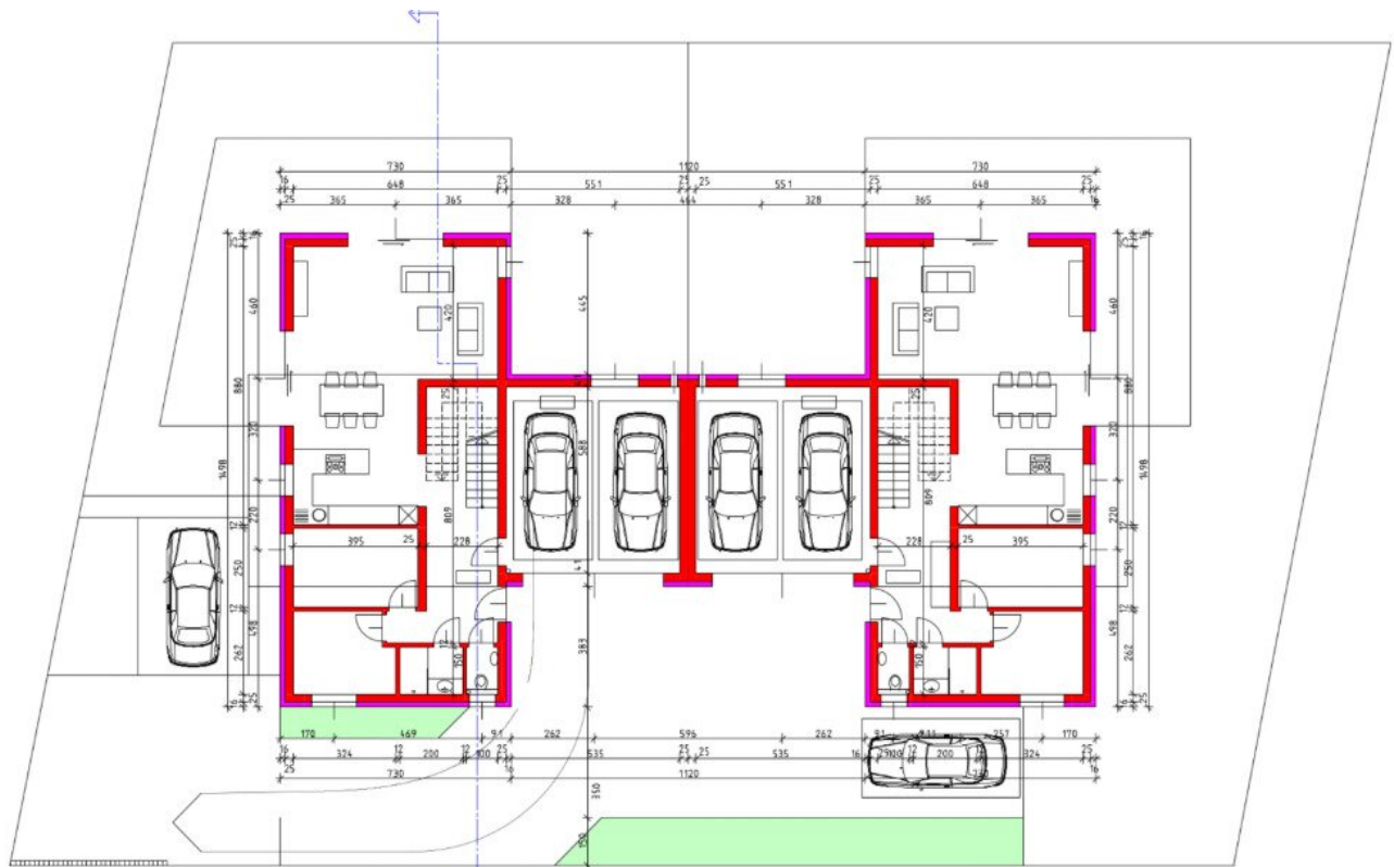
GRUNDRISS EG
