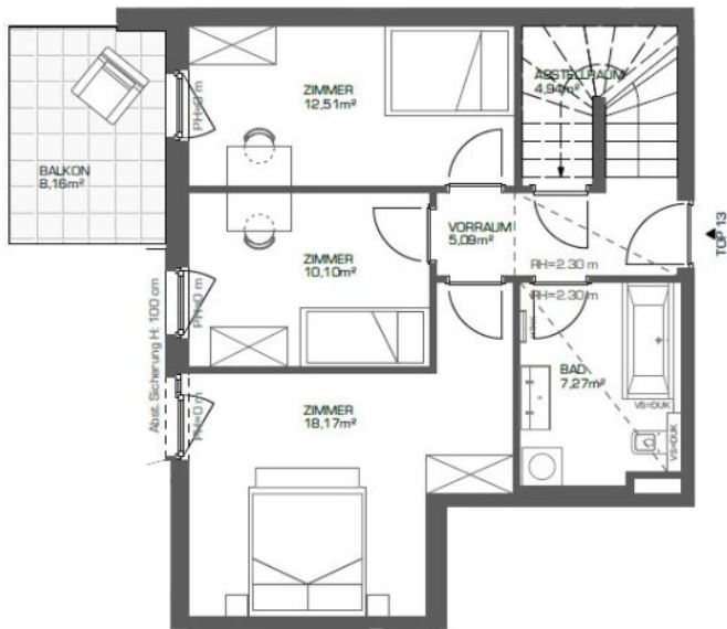
1. Obergeschoss M 1:120
