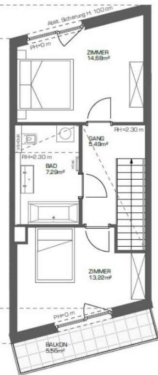
1. Obergeschoss M 1:120
