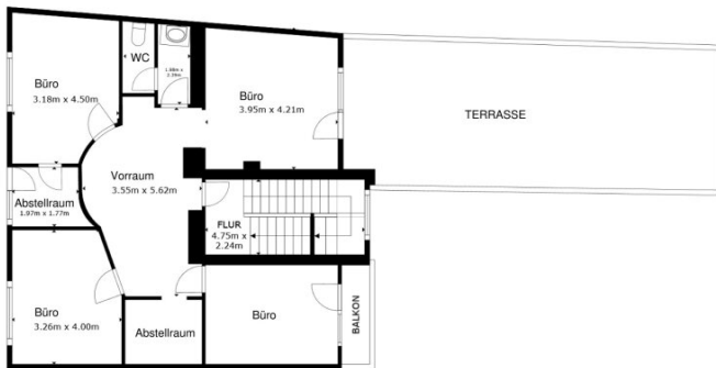
STOCKWERK 1
