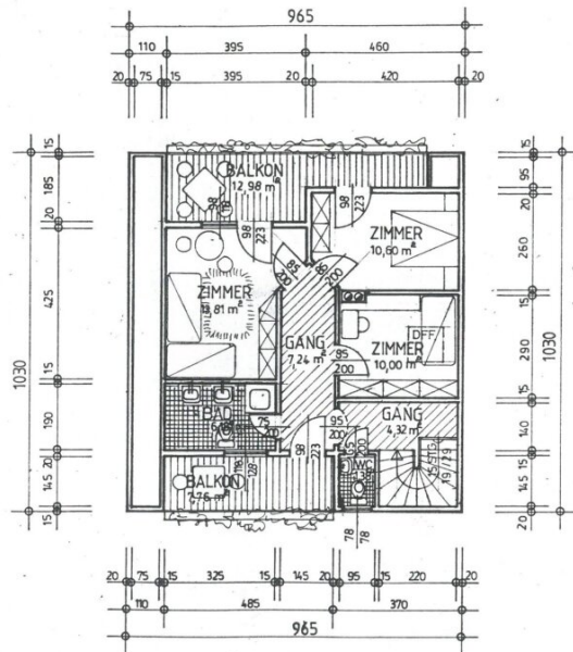
OBERGESCHOSS 1:100
