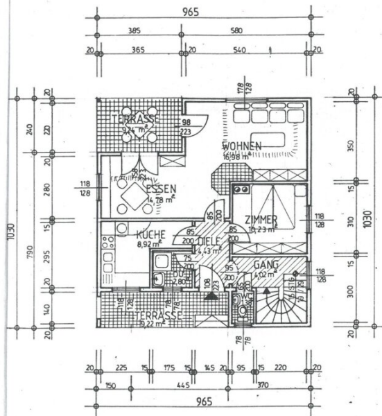
ERDGESCHOSS 1:100
