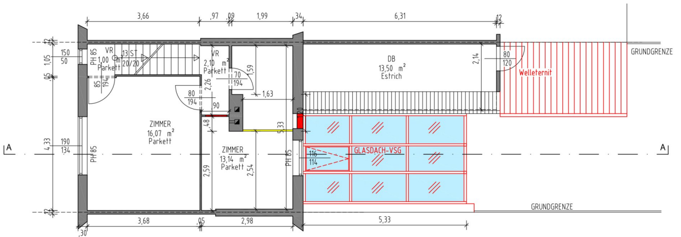
1.OBERGESCHOSS
