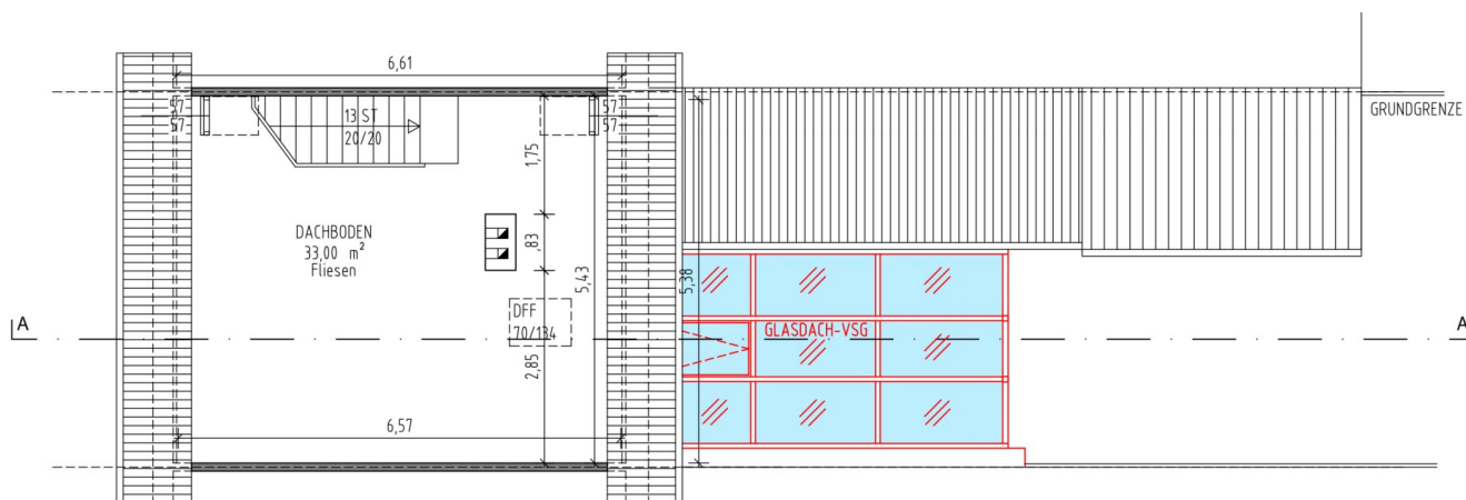
DACHBODEN
