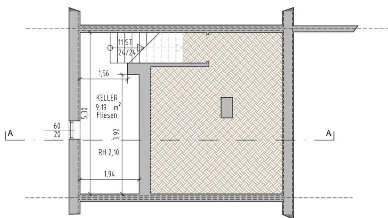
KELLERGECHOSS
