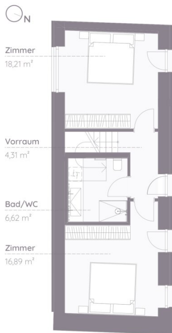
Zwischengeschoß
