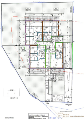
ERDGESCHOSS
