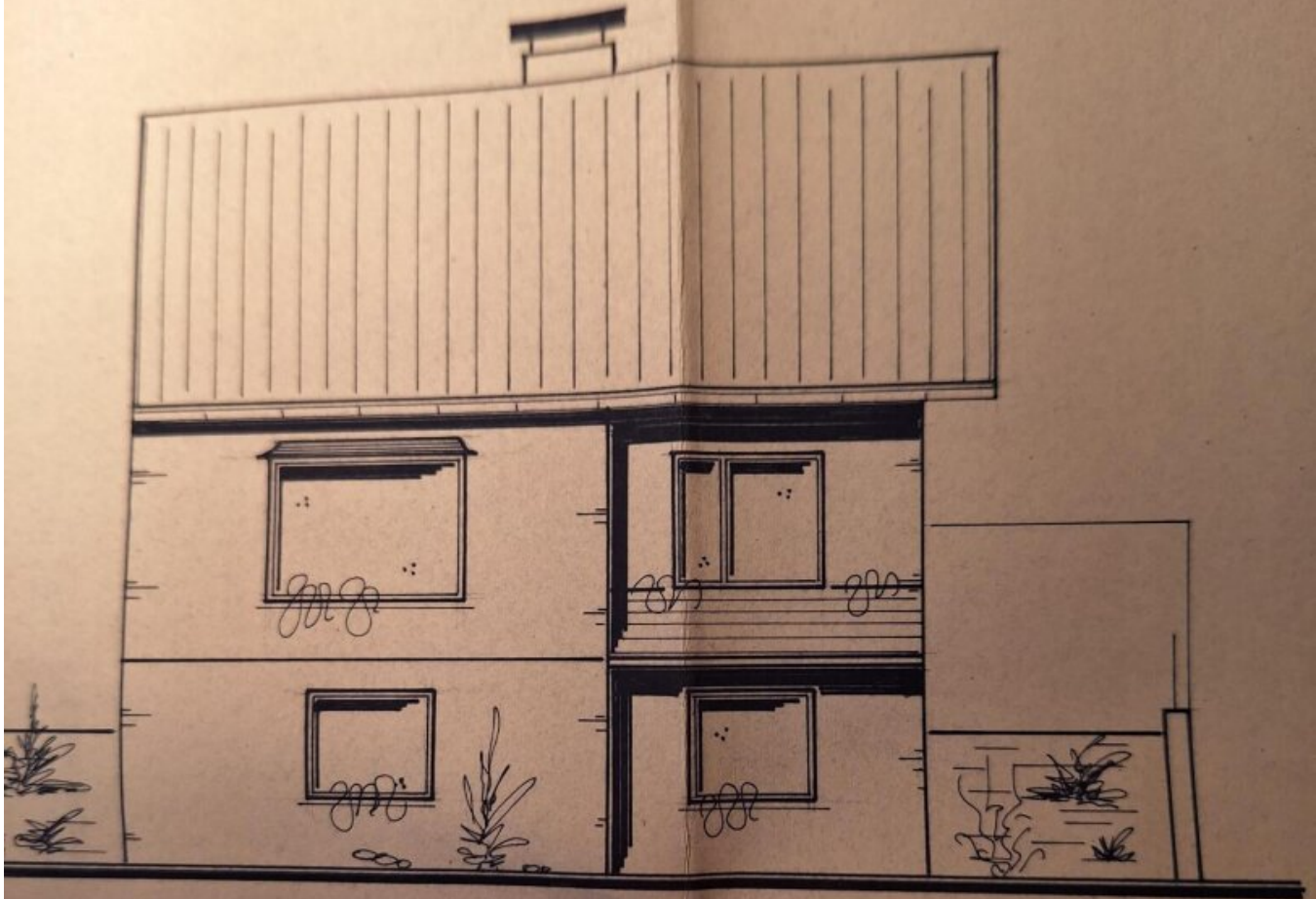
SÜD-ANSICHT
