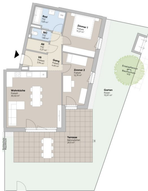
Erdgeschoß
