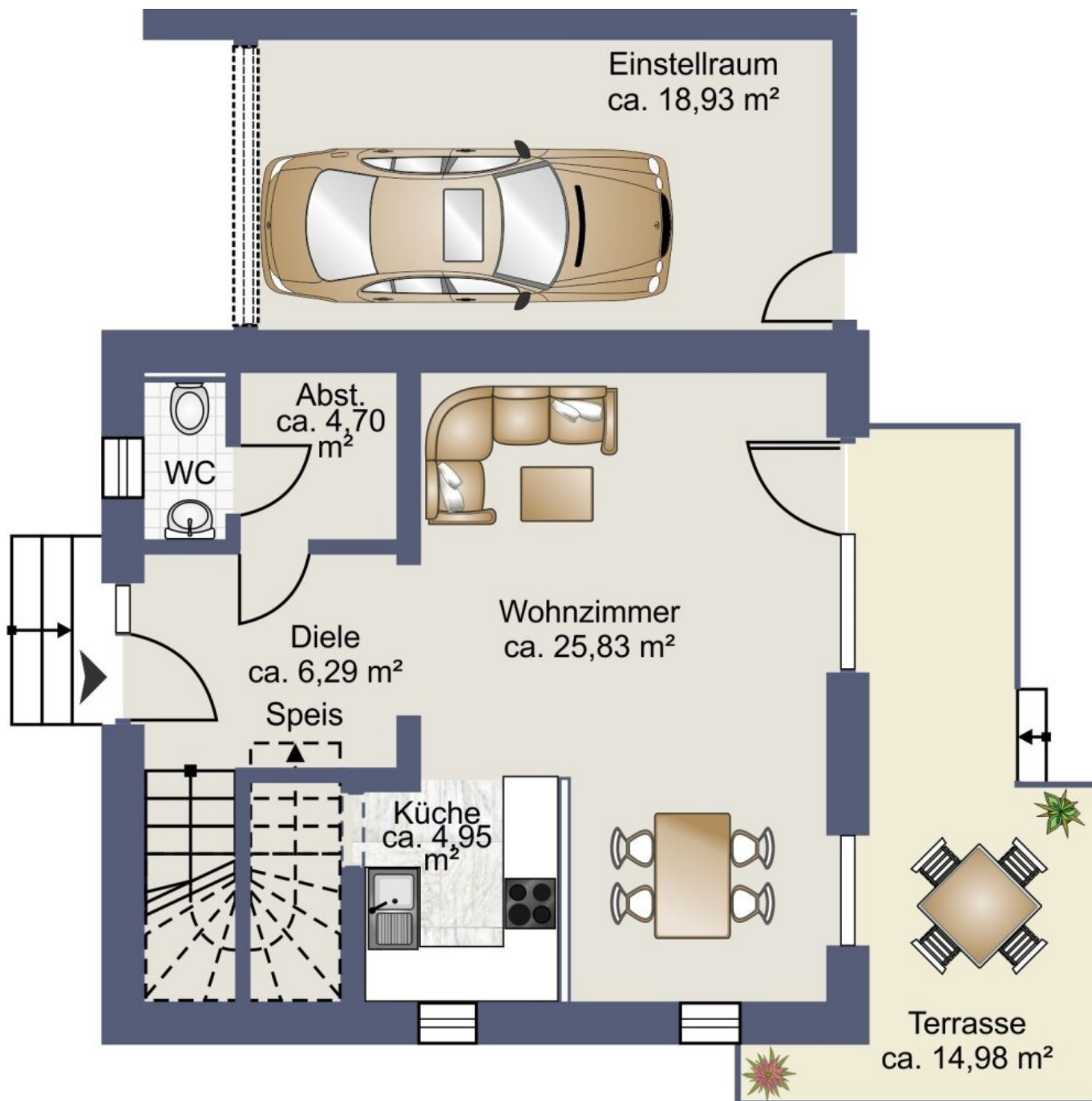
Skizze Erdgeschoss
