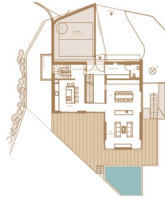
Erdgeschoss
