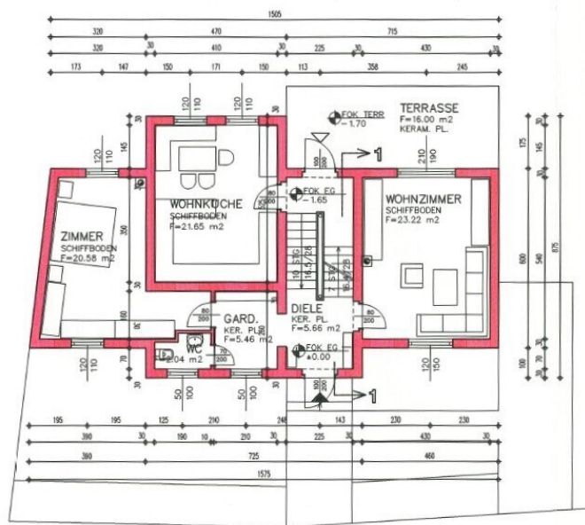
GRUNDRISS ERDGESCHOSS
