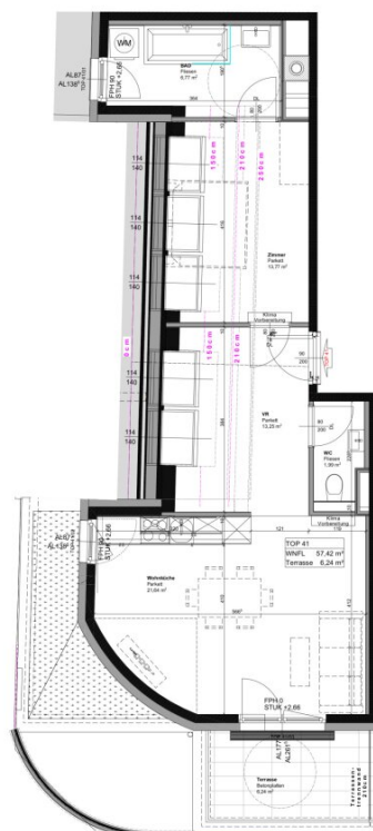
GRUNDRISS 2.DACHGESCHOSS
