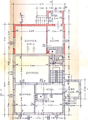
ERDGESCHOSS
