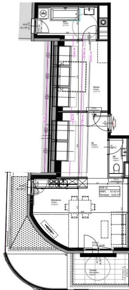
GRUNDRISS 2.DACHGESCHOSS
