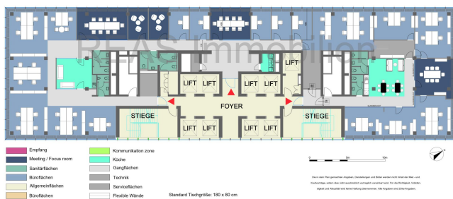
2.OG
