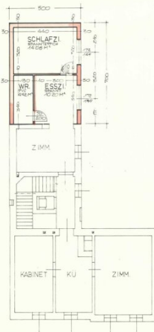
obergeschoss
