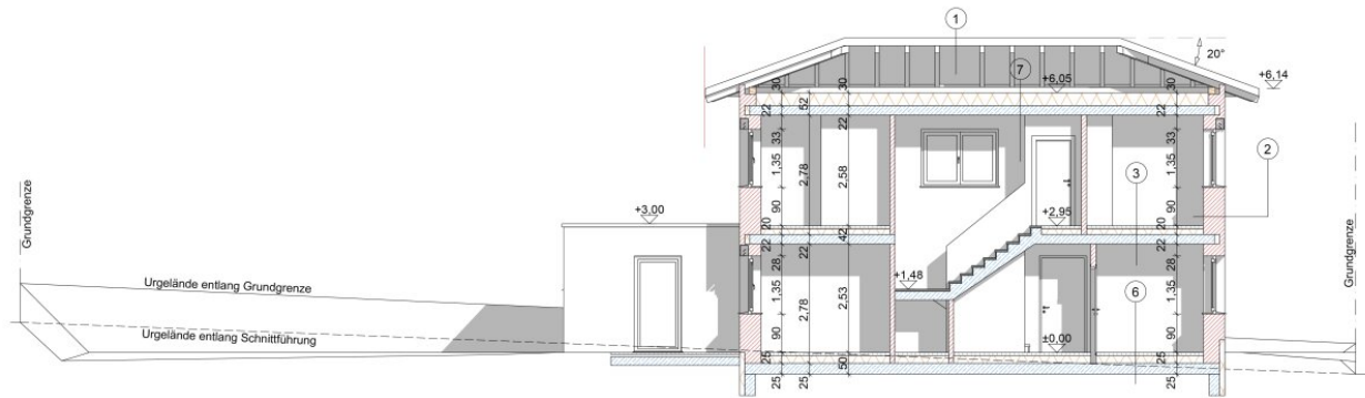
Schnitt A-A
