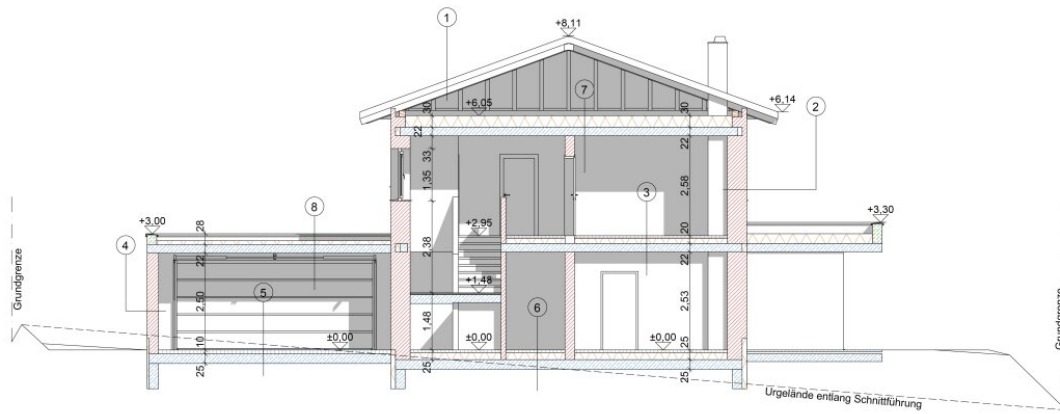
Schnitt B-B
