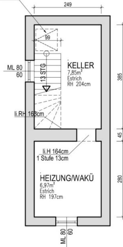
KG 50313 LENZING GRUNDRISS KELLERGESCHOSS 1:100 7.4.2024 / mm
