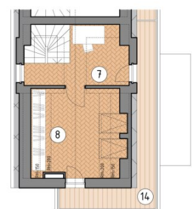
2. Obergeschoss
