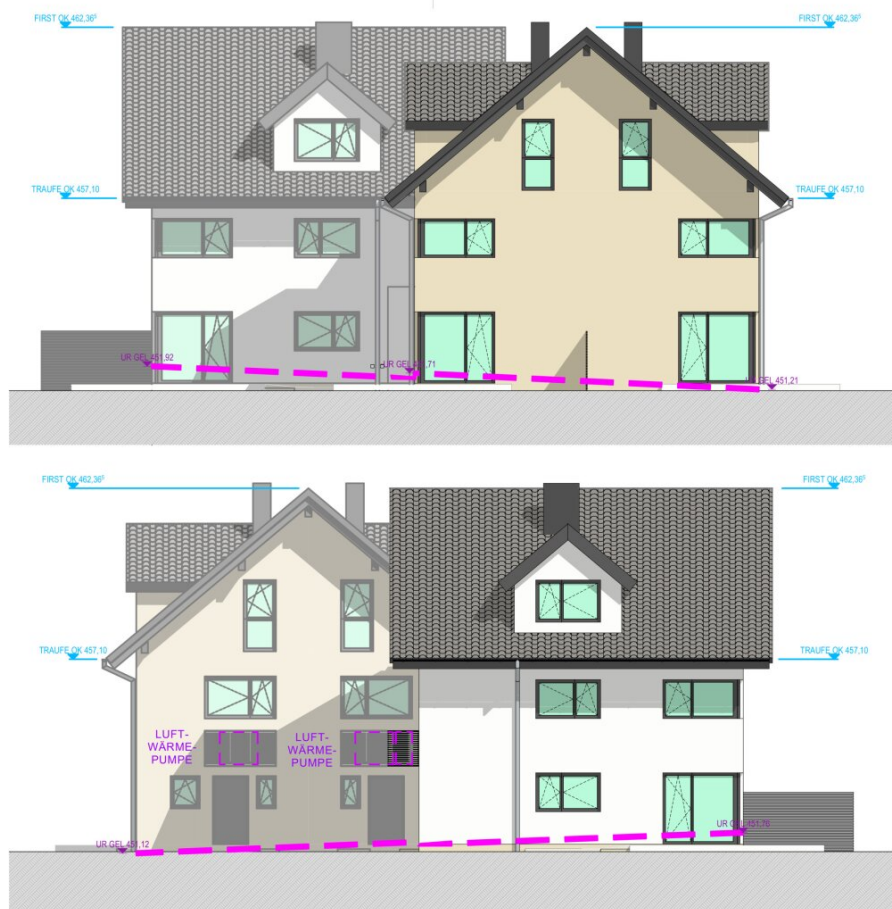
OSTANSICHT
