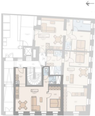
EG Etagengrundriss
