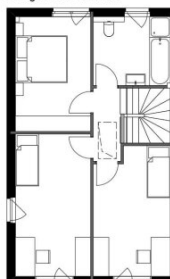
Obergeschoss TOP 5.1
