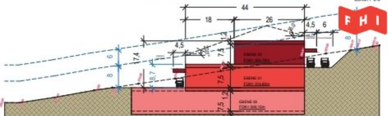
SCHNITT B-B
