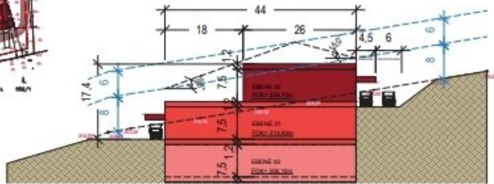
SCHNITT C-C
