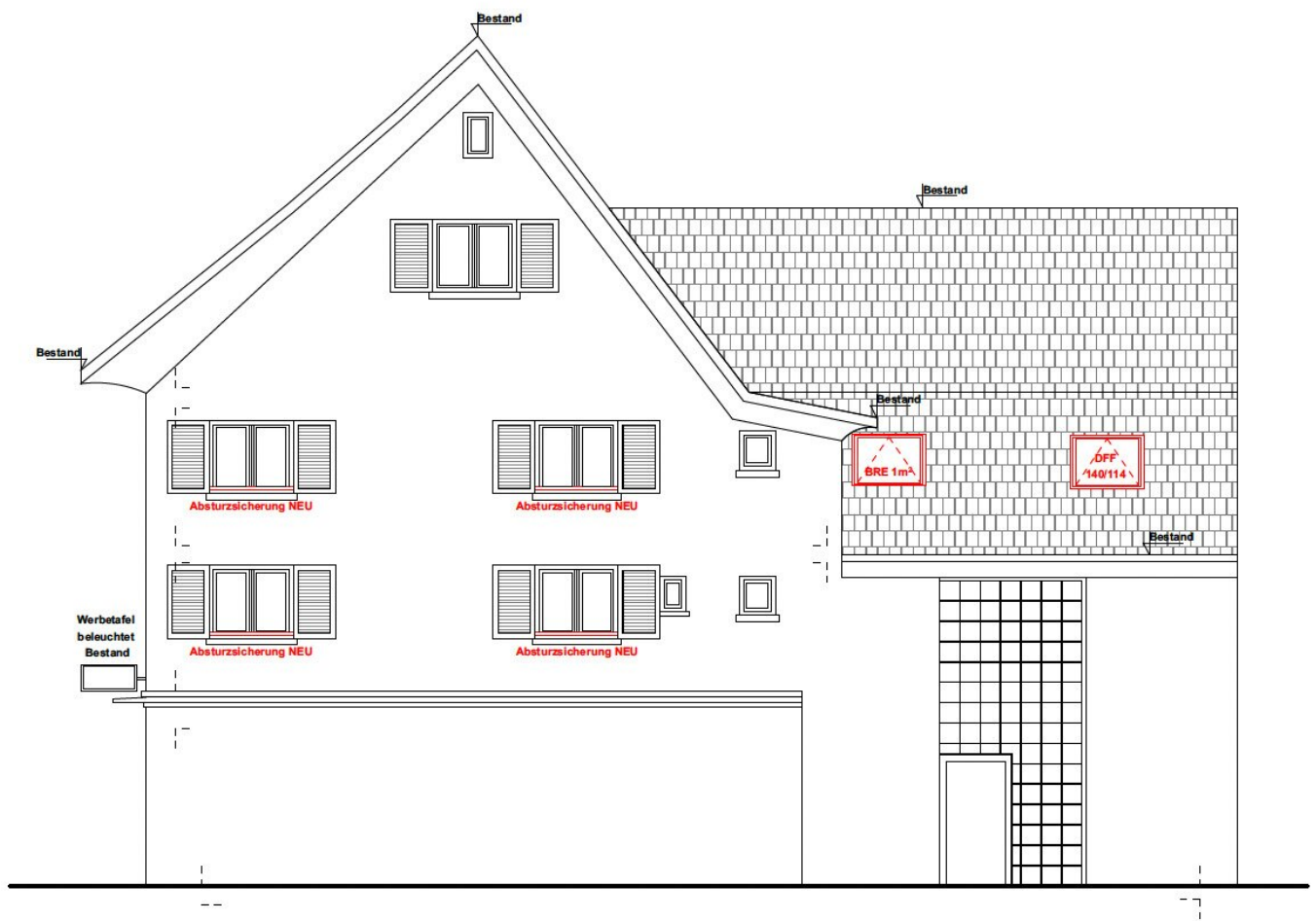
Nordansicht
