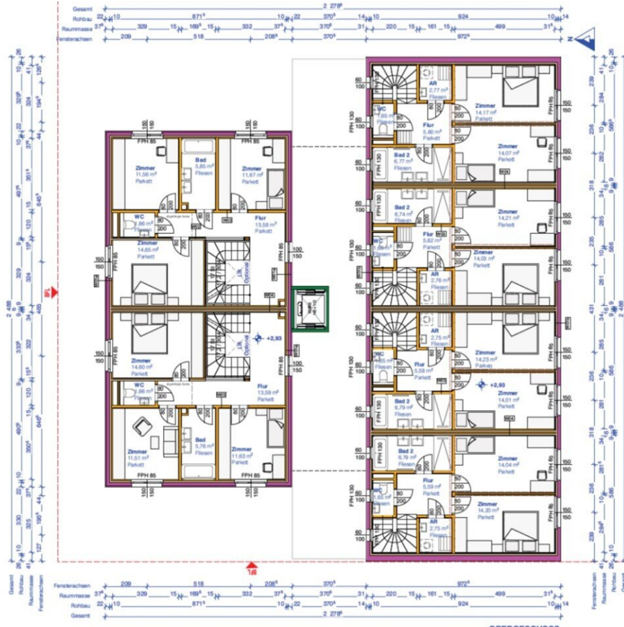
OBERGESCHOSS 1:100
