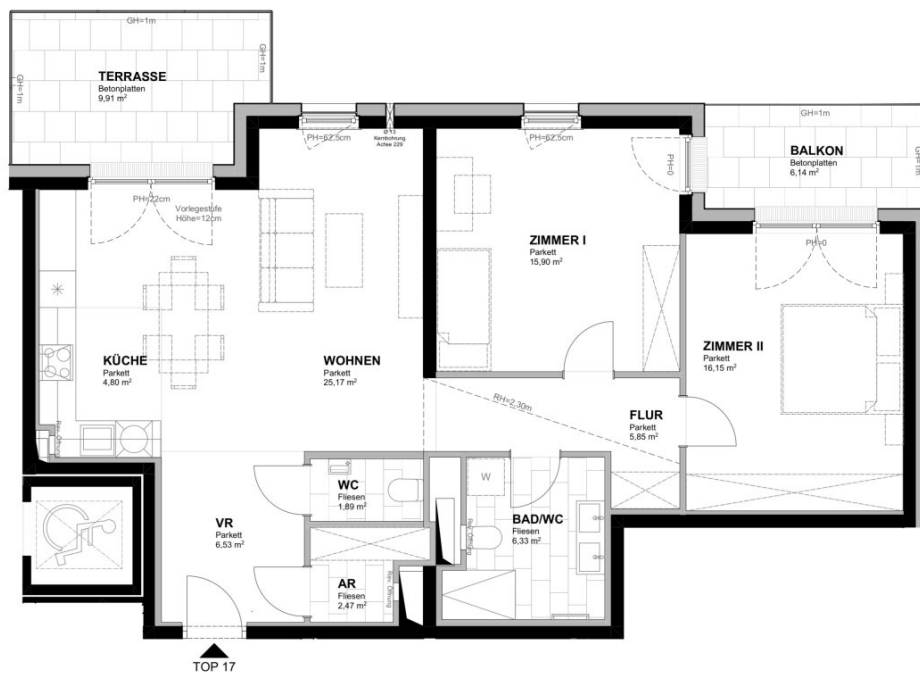
Übersichtsplan Dachgeschoss
