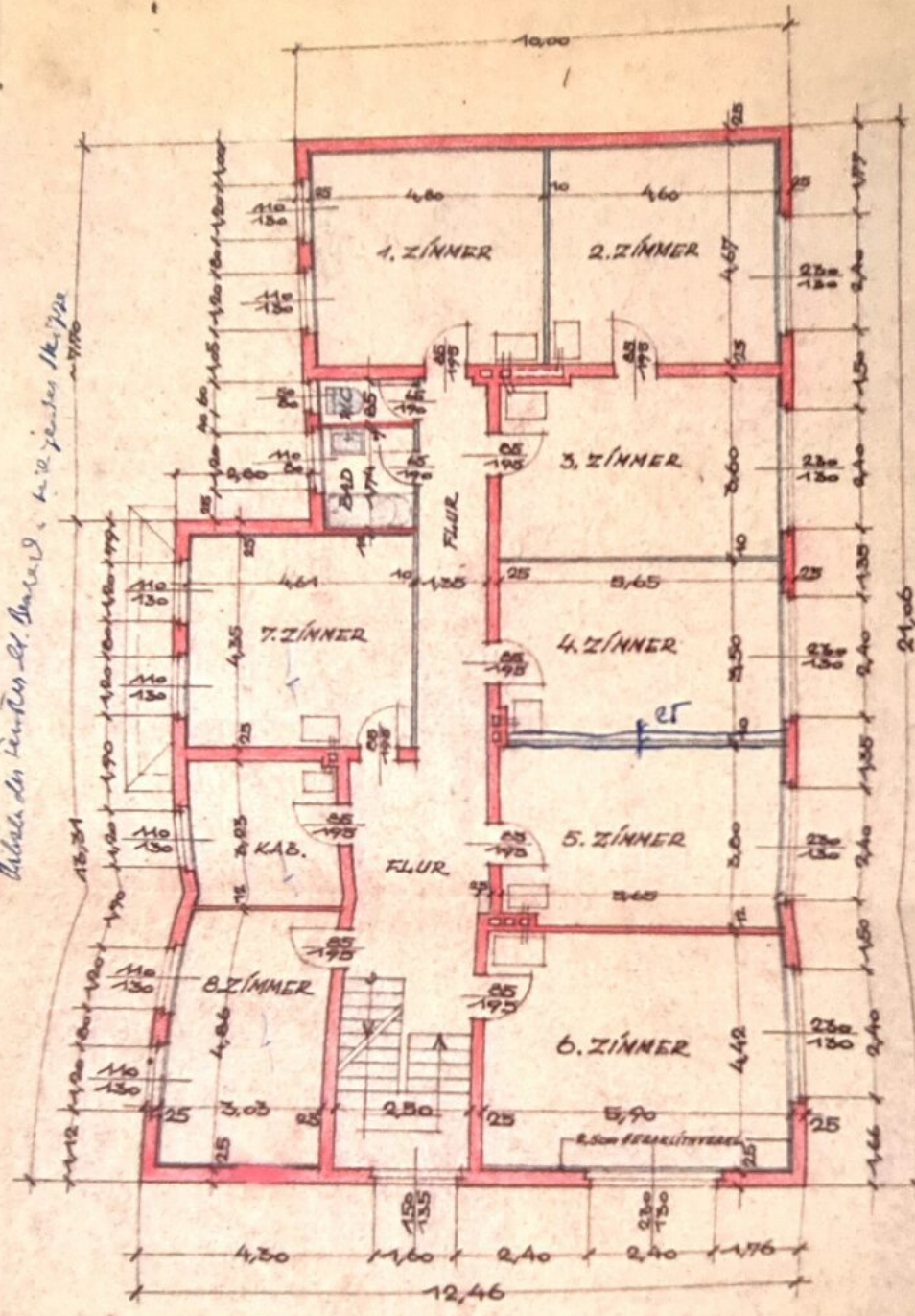
OBERGESCHOSS - GRUNDRISS
