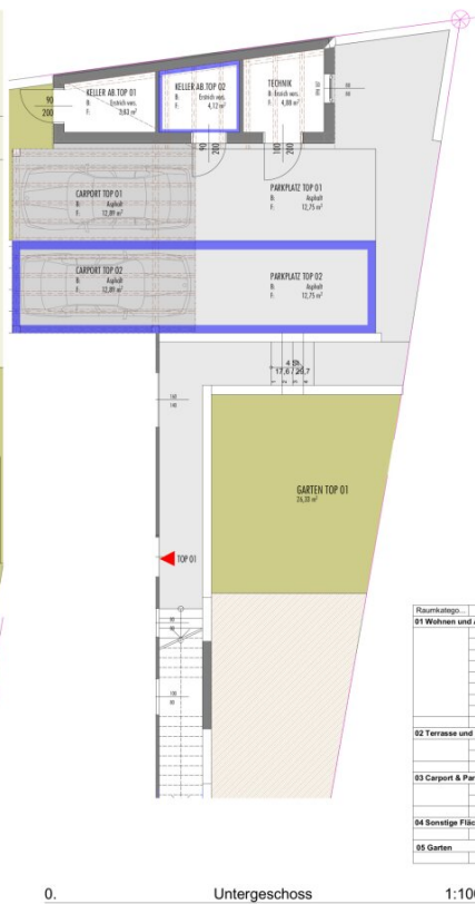
0. Untergeschoss 1:100
