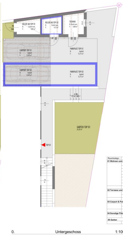
0. Untergeschoss 1:100
