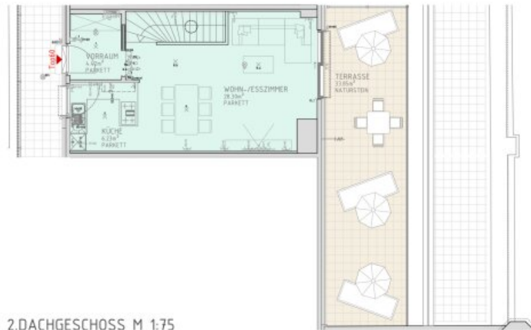
2.DACHGESCHOSS M 1:75
