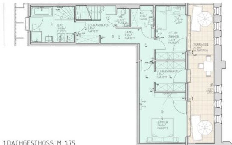
1.DACHGESCHOSS M 1:75
