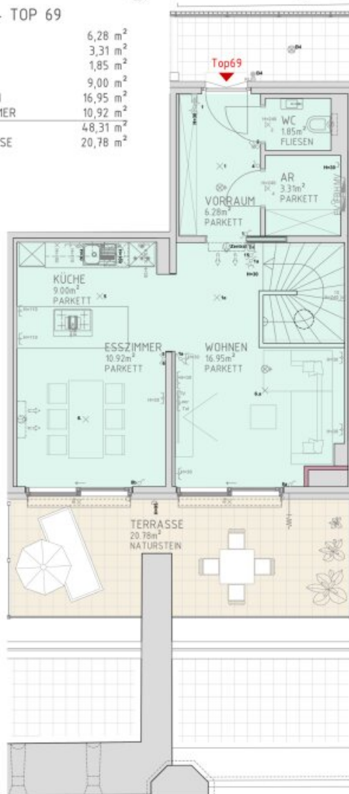
2.DACHGESCHOSS M 1:50
