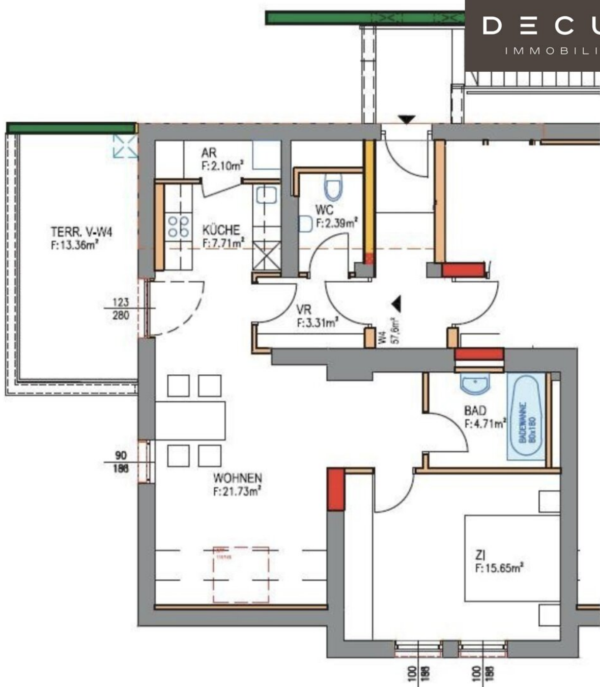
GRUNDRISS DG VILLA - WOHNUNG 5:
